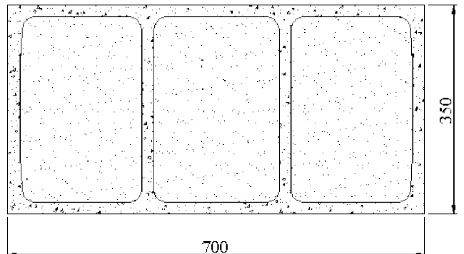
CASETÓN DE 70 – Canto 350mm.
