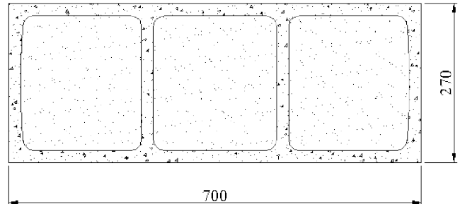
CASETÓN DE 70 – Canto 270mm.
